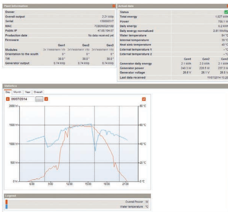
Bild 3: Monitoring der Energieerträge in »AE SiteLink«.
